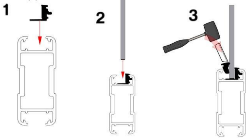
For dør på langsiden
