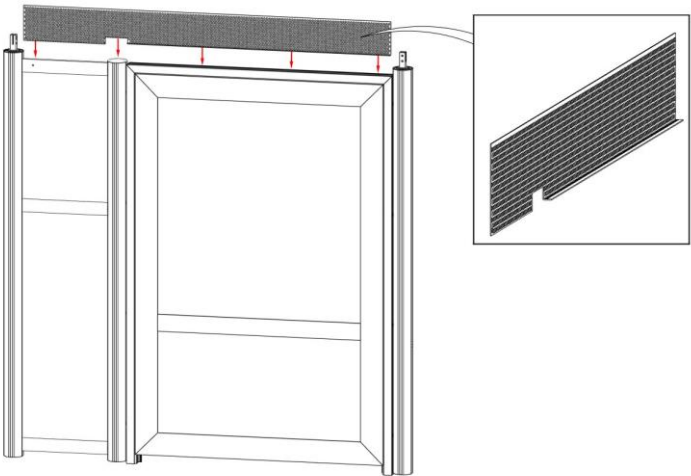
For dør på langsiden
