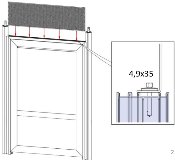
For dør på gavlside
